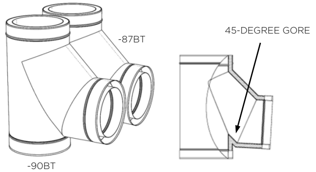
Figure 4-4, 87° & 90° Boot Tee (__BT)
